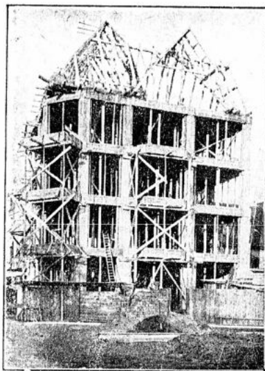
Geschäfts- und Wohnhaus in Guben i. L. (Ganz in Eisenbeton ausgeführt 1908.) Rohbau.
